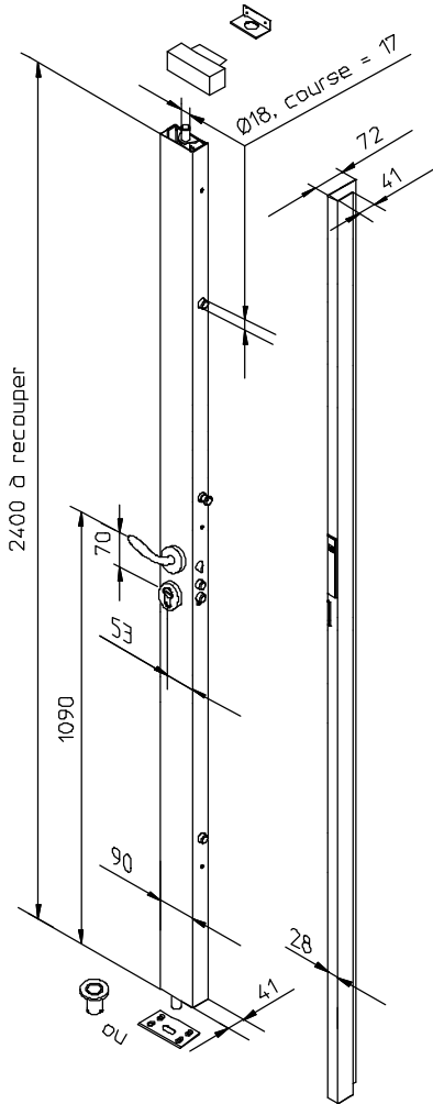
gâche standard monobloc en J
