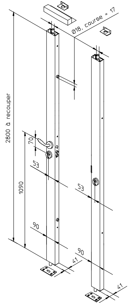
2 vantaux 2800 mm
